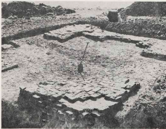
Vlaardingen, Holy (25), de 4 hoekpijlers van de fundering, de tussenruimte rechtsachter is gevuld met metselwerk uit circa 1600.
